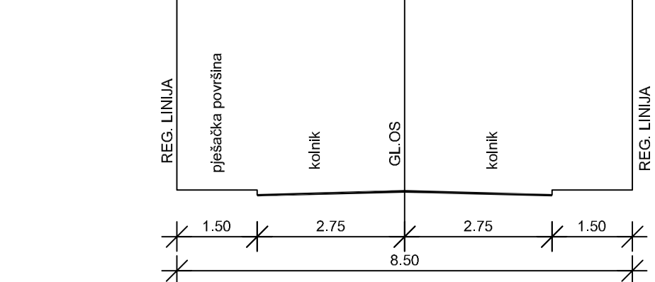
POPREČNI PRESJEK "B"
