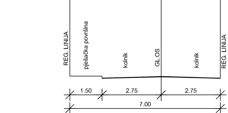
POPREČNI PRESJEK "C"
