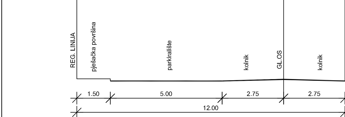
POPREČNI PRESJEK "A"
