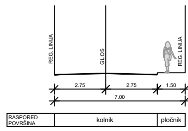
POPREČNI PRESJEK "B"
