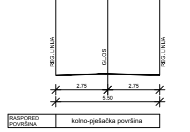
POPREČNI PRESJEK "C"
