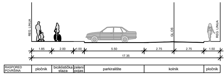
POPREČNI PRESJEK "A"
