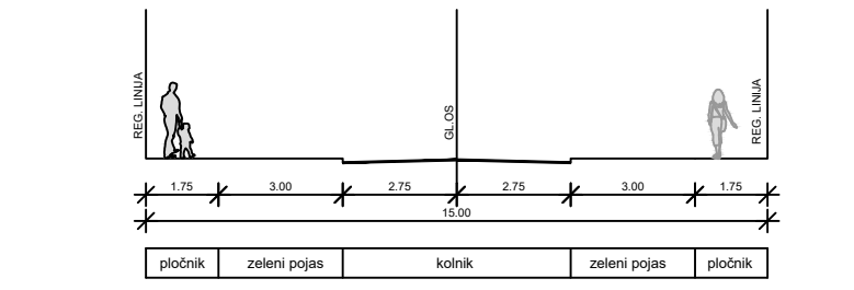
POPREČNI PRESJEK "D" - cesta s posebnim režimom korištenja
