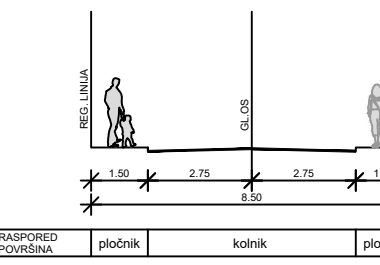
POPREČNI PRESJEK "E"
